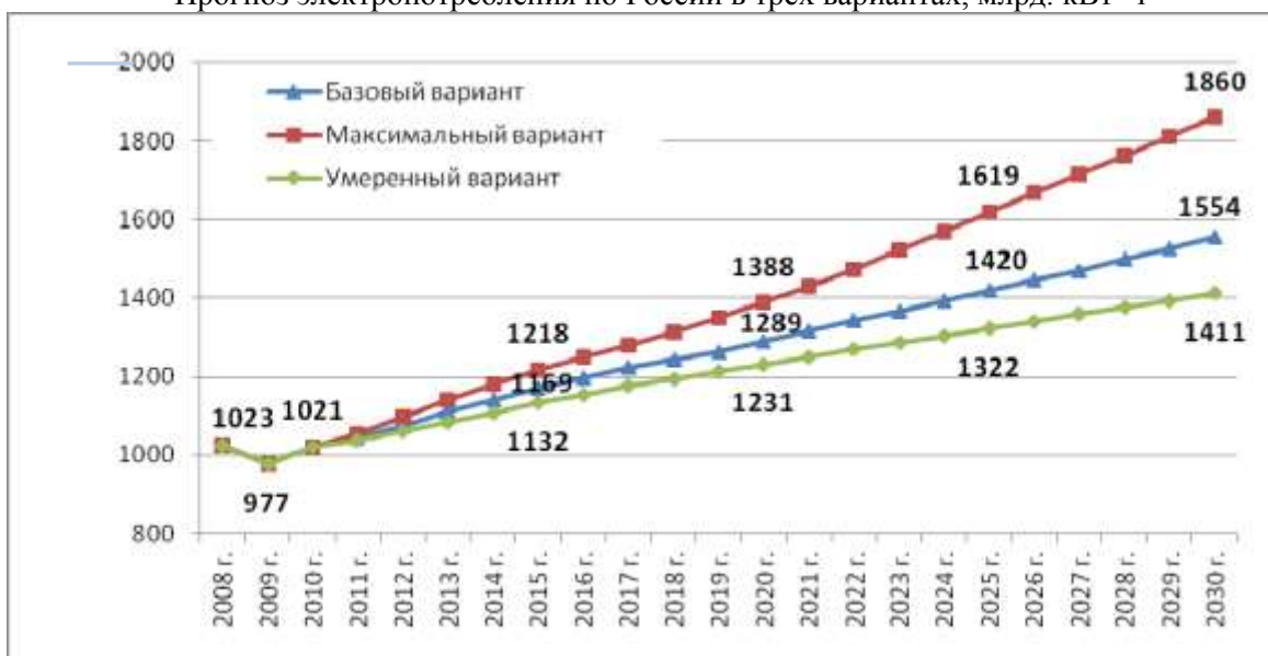
Прогноз электропотребления по России в трех вариантах, млрд. кВт*ч
